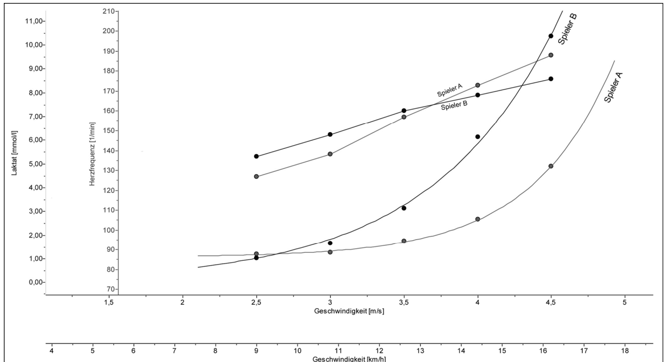
Abb.1: Feldstufentest
